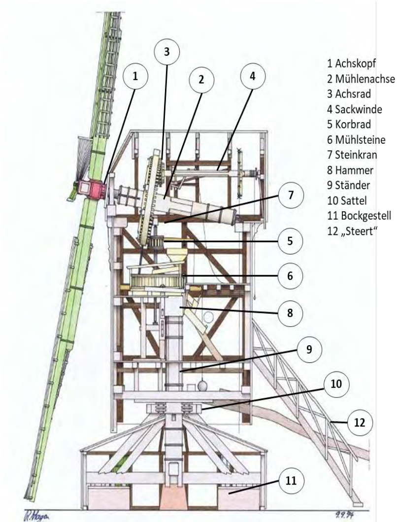
Abbildung 3 Aufriss einer Bockwindmühle
